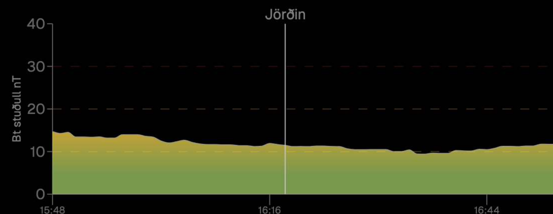
Sviðsstyrkur (Bt)
